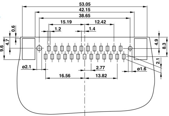
25 Way
