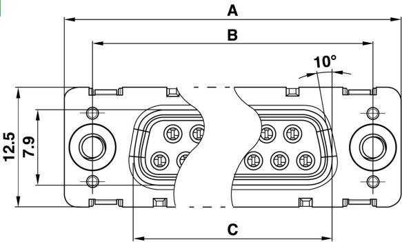
Socket
